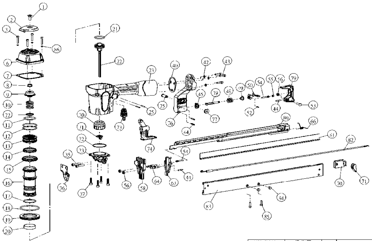
SN50S5LM.B01 爆炸图 D 2018/06/04
